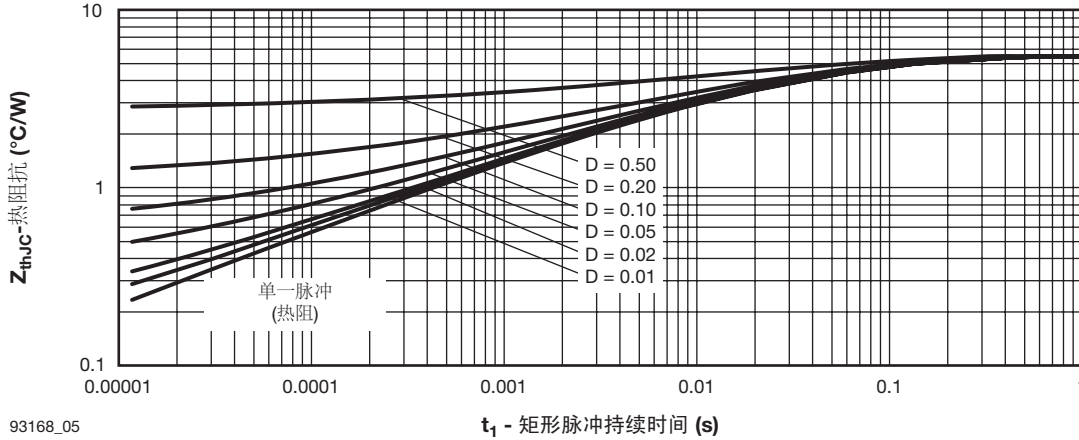
图 5. 最大热阻抗 Z_{thJC} 特性图 (FULL-PAK)
