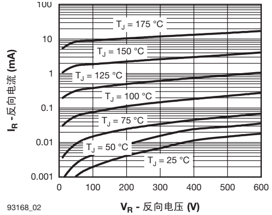
图 2. 反向电流与反向电压典型值
