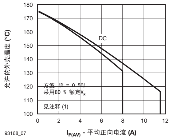
图 7. 允许的最大外壳温度和平均正向电流的关系图 (FULL-PAK)
