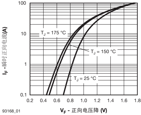
图 1. 典型正向压降特性
