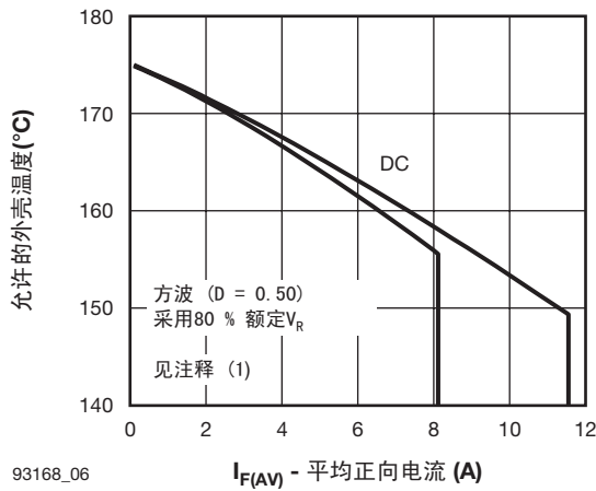
图 6. 允许的最大外壳温度和平均正向电流的关系图 (TO-220)
