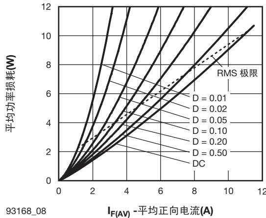
图 8. 正向功率损耗特性
